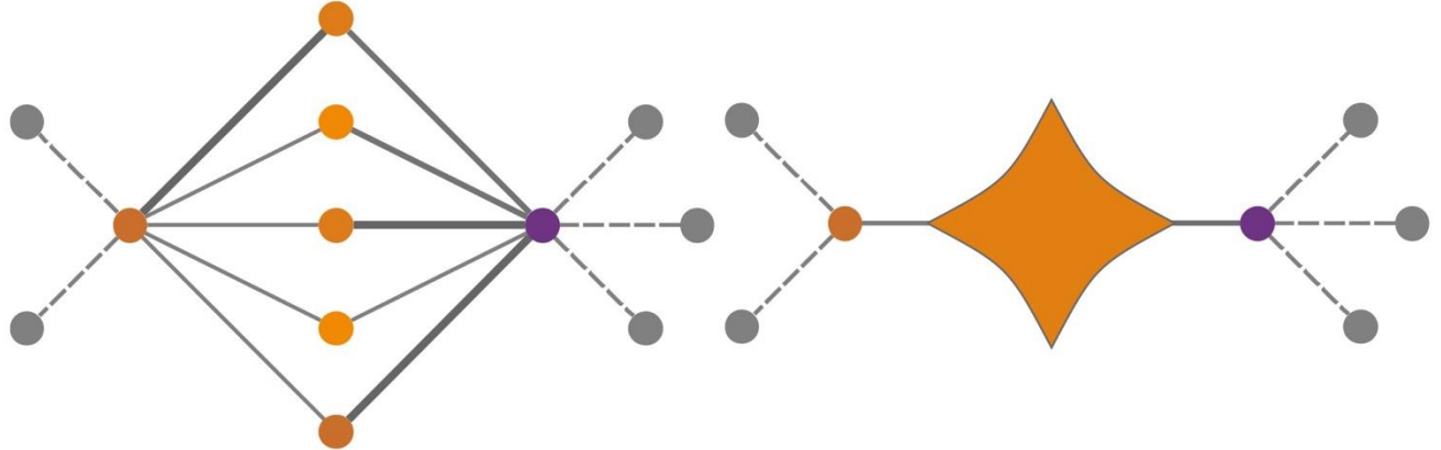
Fan
