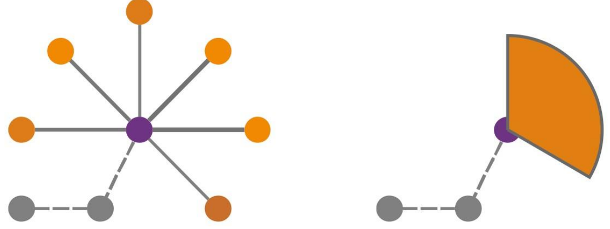
Fan
